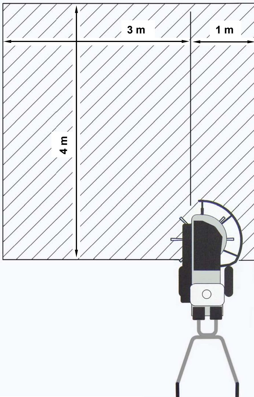
Abbildung 1 : Gefahrenbereich
