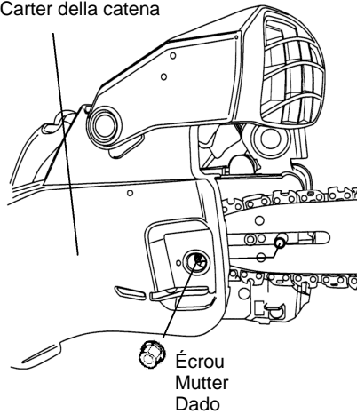
Fig.1 Carter de chaîne Kettenkasten Carter della catena
