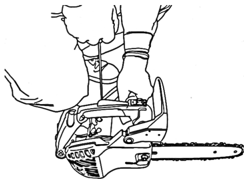
Bouton de l'enrichisseur Luftklappenknopf Manopola dell'avviamento (Starter)
