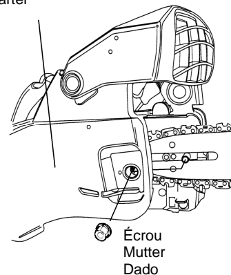
Carter de chaîne Kettenkasten Carter
