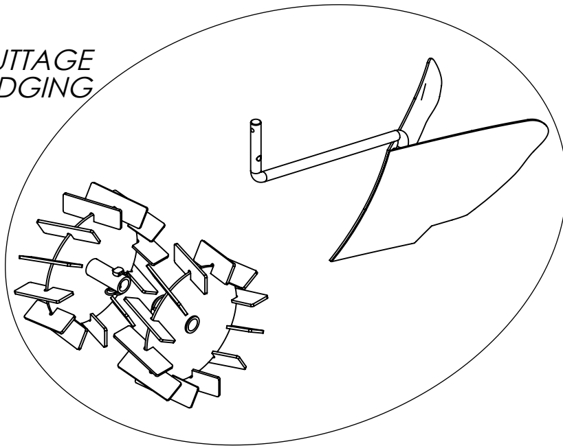
EMOUSSEUR LAWN DETACHER
