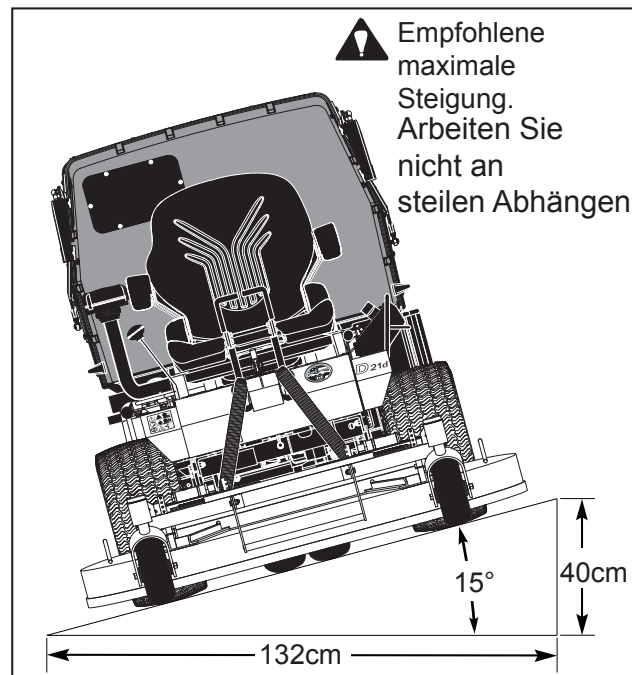
Maximale Seitenneigung
