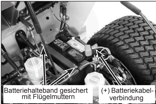
Batteriemontage
