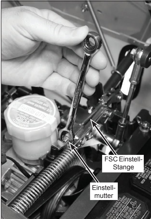
Einstellung der Neutralfunktion
