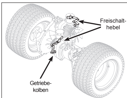
Position Getriebefreischalthebel
