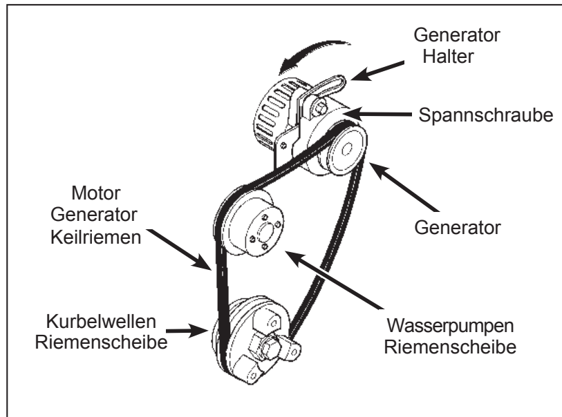
Motor Generator-Keilriemen (gelockert)
