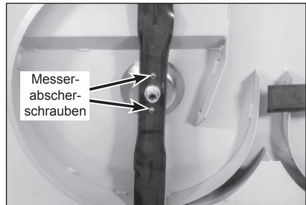
Mähmesser Scherschrauben
